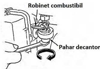
Robinet combustibil
